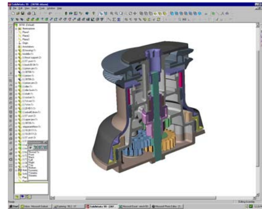
Vista esplosa ed in sezione di un Verricello
