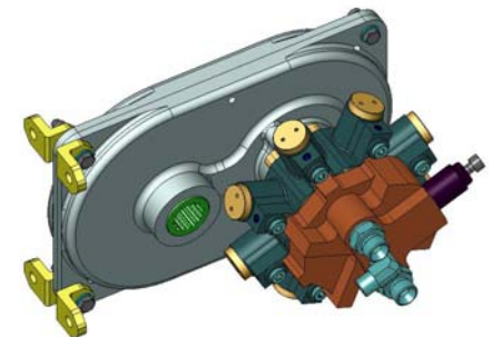
Pompa manuale ad 8 cilindri con riduttore per coffee grinder
