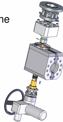
Valvola automatizzata per centrale idroelettrica
